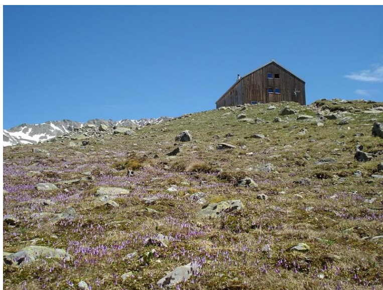
Keschhütte: Tagesziel am 1. Tag
